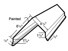
LG 126 DOOR POST TRIM*
